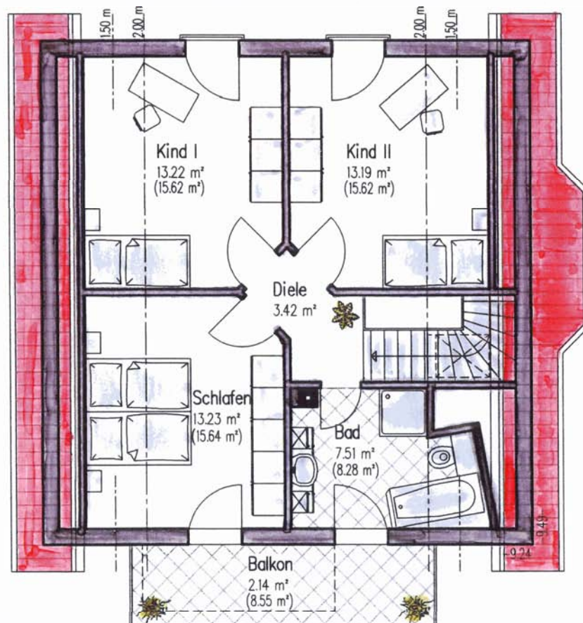
Dachgeschoss M 1:100
