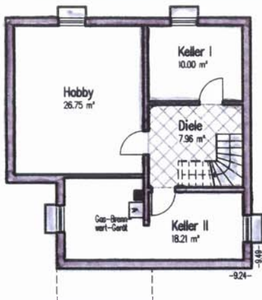
Kellergeschoss M 1:200
