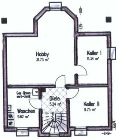
Kellergeschoss M 1:200
