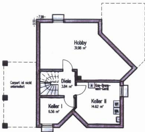
Kellergeschoss 1:200
