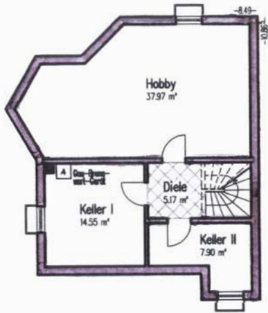
Kellergeschoss M 1:200
