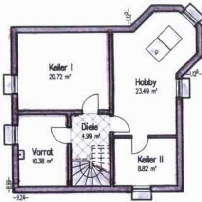
Kellergeschoss M 1:200
